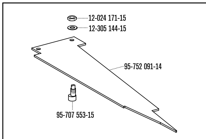
95-752 091-13 (Für gebogene Abnäher) (For curved darts) (Pour pinces curbes) (Para pinzas curvadas)
